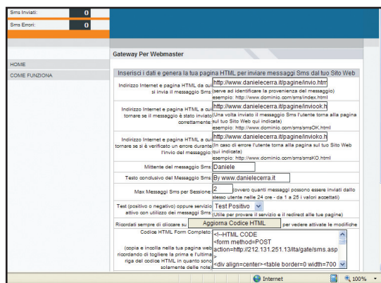
Figura 2 - L'impostazione dei dati di configurazione del Gateway SMS per il nostro sito richiede pochi rapidi passaggi
